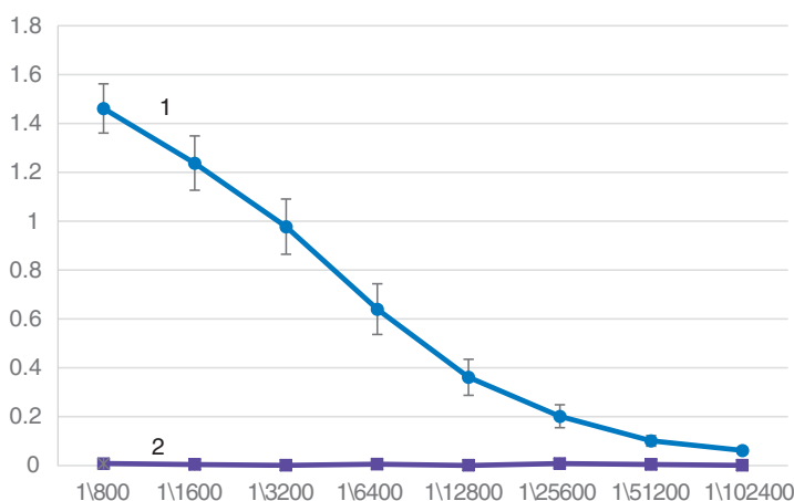
Рис. 1. Уровень антител к вирусу гриппа A/Chicken/NJ/294598-12/2004-MA (H7N2) в сыворотках крови мышей, иммунизированных аденовирусом Ad5-tet-M2NP. Ось ординат — оптическая плотность (OD); ось абсцисс — разведение сыворотки. (1) опытная группа; (2) контрольная группа. Значения OD опытной группы достоверно выше контрольной, p < 0,001 .
