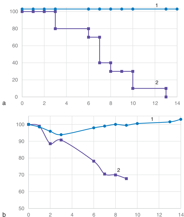
Рис. 2. Защитные свойства иммунизации мышей рекомбинантным аденовирусом Ad5-tet-M2NP от заражения 5 LD 50 вируса гриппа A/Chicken/NJ/294598-12/2004-MA (H7N2). а — динамика выживаемости. Ось ординат — количество выживших животных, %; ось абсцисс — продолжительность, сут. б — динамика снижения массы тела. Ось ординат — изменение массы тела животных, % от исходной; ось абсцисс — продолжительность, сут. (1) опытная группа; (2) контрольная группа. Достоверная разница между выживаемостью в опытной и контрольной группах p < 0,0001 , между изменением массы тела в опытной и контрольной группах p < 0,05 .
