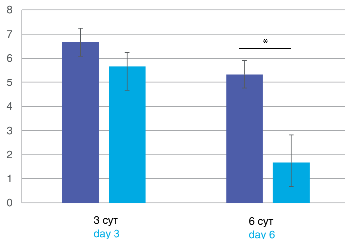
Рис. 3. Титры вируса гриппа A/Chicken/NJ/294598-12/2004-MA (H7N2) (среднее значение Ig(TCID 50 )) в легких мышей, иммунизированных рекомбинантным аденовирусом Ad5-tet-M2NP, после заражения вирусом гриппа A/Chicken/NJ/294598-12/2004-MA (H7N2). (■) контрольная группа; (■) опытная группа. * p < 0,05 .
